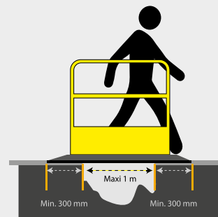
FIXATION POSSIBLE AU SOL Perçage aux 4 coins
